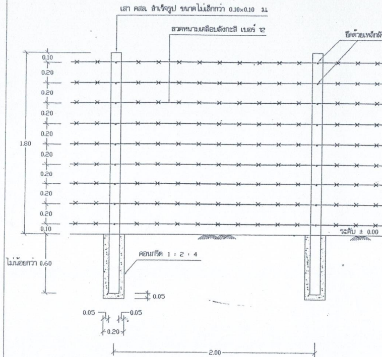
รูปด้านรื้อลวดหนาม 1:20
