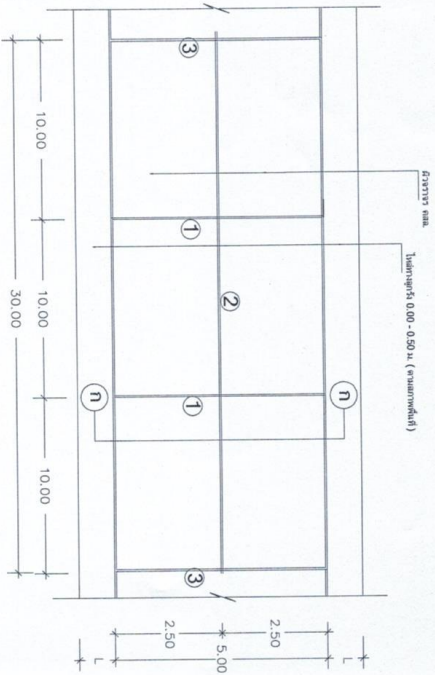
แปลนการวางเหล็ก TIE BAR SCALE NONE
